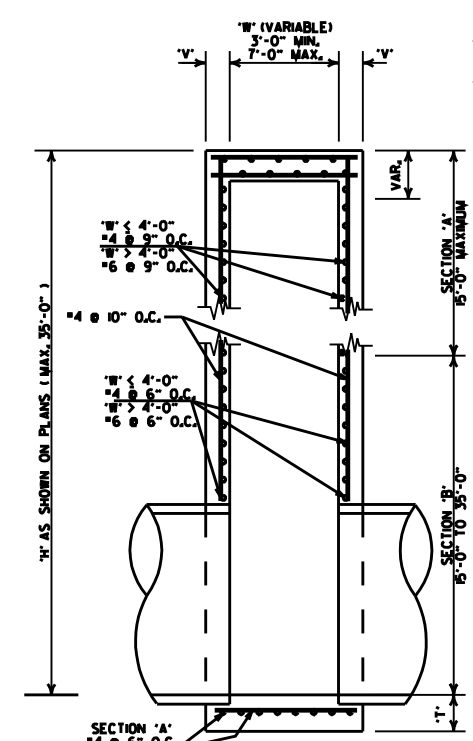
SECTION A-A
